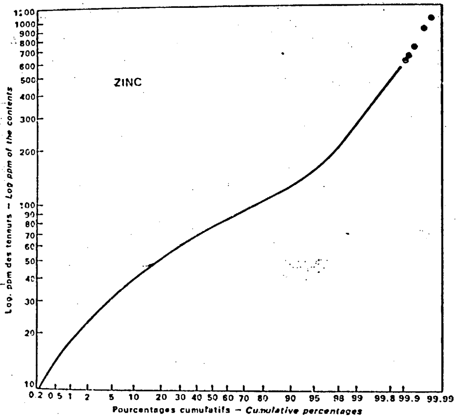
Courbes de fréquences cumulatives des teneurs (sur papier gaussien - logarithmique)
