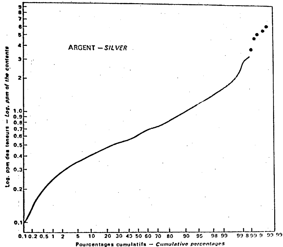
Courbes de fréquences cumulatives des teneurs (sur papier gaussien - logarithmique)
