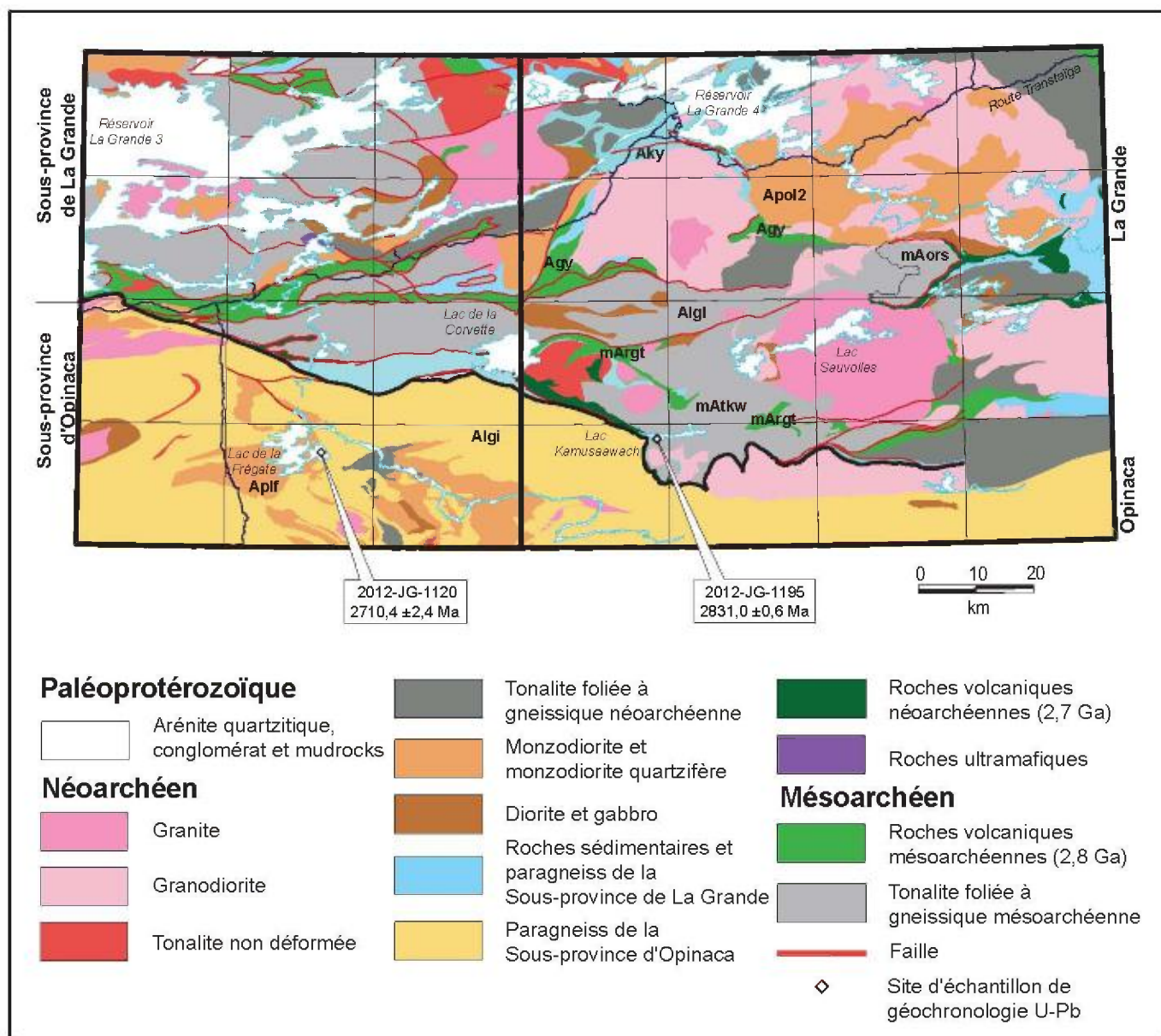
FIGURE 3 – Géologie simplifiée des feuillets SNRC 33G et 33H et localisation des sites d'échantillonnage de géochronologie (Algi : Complexe de Langelier; mAors : Intrusion d'Orsigny; mAtkw : Intrusion de Kamusaawach; Apol : Batholite de Polaris; Apif : Pluton de la Frégate; Algi : Complexe de Laguiche; Aky : Formation de Keyano; mArgt : Formation de Rouget; Agy : Groupe de Guyer).
