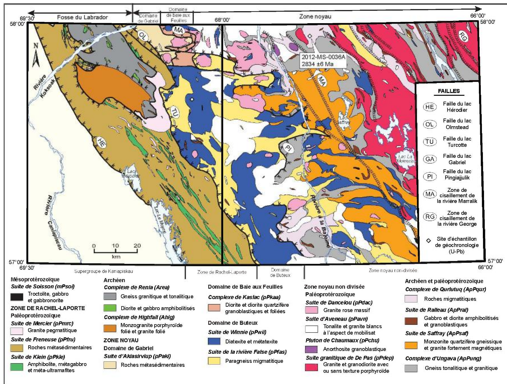
FIGURE 1 – Géologie simplifiée de la région du lac Saffray (feuillets SNRC 24F et 24G), Province de Churchill, et localisation du site d'échantillonnage de géochronologie.
