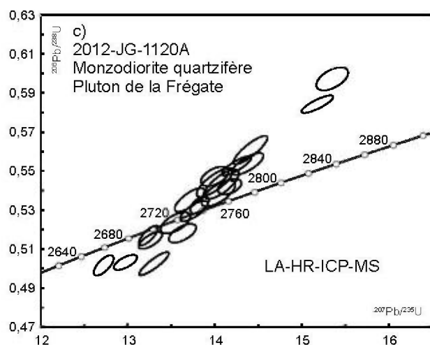
FIGURE 9 – Diagrammes concordia et diagramme de probabilité cumulative (figure 9d) des analyses de zircons pour les échantillons en provenance des sous-provinces de La Grande et d'Opinaca effectuées par les méthodes ID-TIMS et LA-HR-ICP-MS. Les résultats analytiques sont présentés aux tableaux 2 et 3
