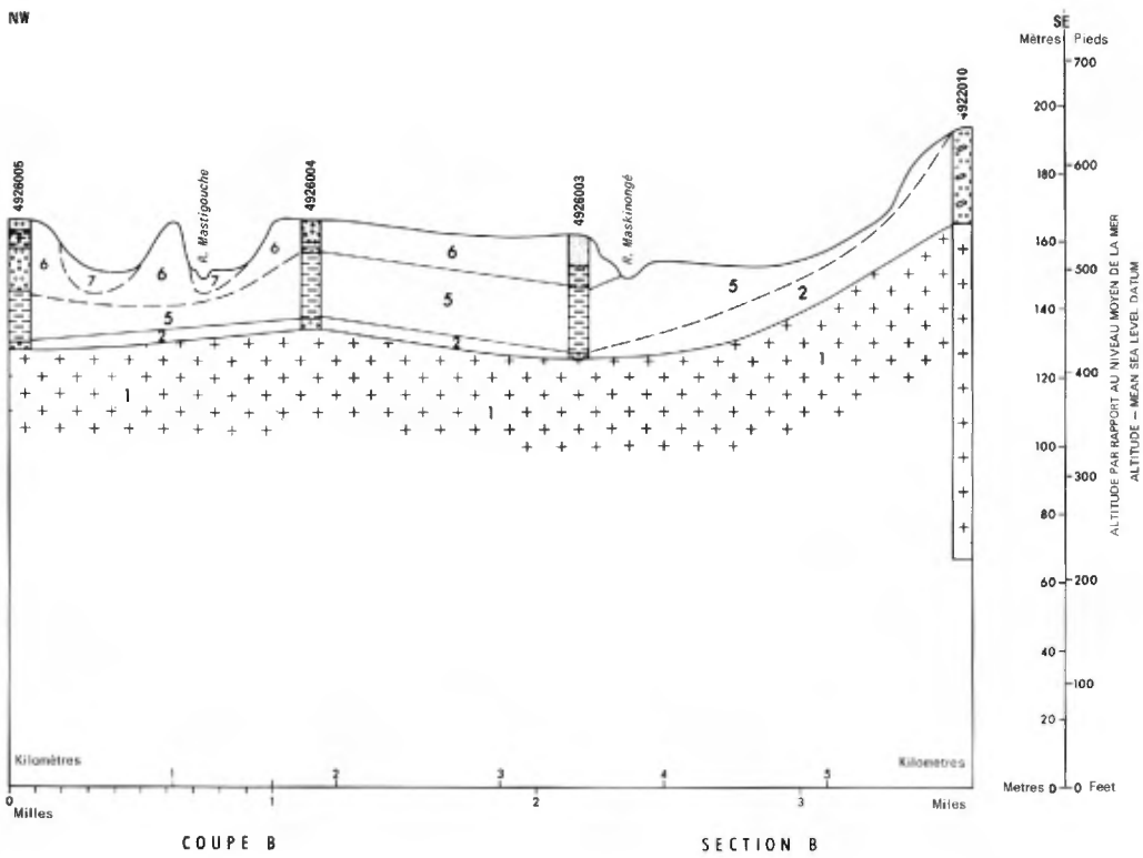
FIGURE 26 - Coupes géologiques A et B./Geological sections A and B.
