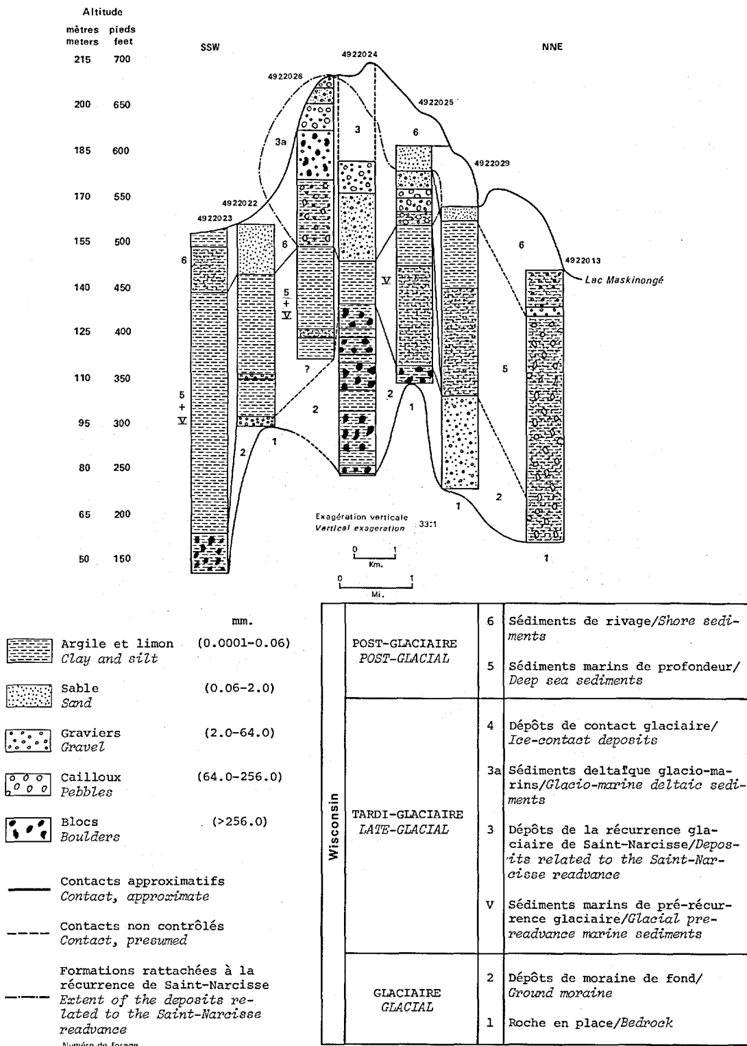
FIGURE 13 - Coupe transversale de la moraine terminale de Saint-Narcisse. à Saint-Gabriel. Voir aussi la figure 27. Section through the Saint-Narcisse terminal moraine at Saint- Gabriel. See also figure 27.
