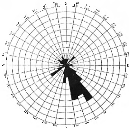
FIGURE 11 - Directions des plongées de cailloux. Moraine de Saint-Narcisse à Saint-Gabriel (100 mesures). Dip directions of pebbles - Saint-Narcisse terminal moraine, at Saint-Gabriel (100 measurements).
