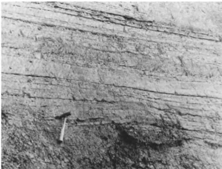
Pl. X-B - Argiles stratifiées dans une coupe à environ 2 milles au nord-ouest de Saint-Siméon. Stratified clays in roadcut about 2 miles northwest of Saint-Siméon.
