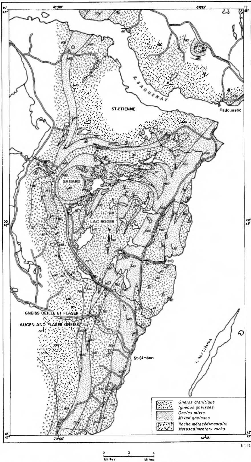
Figure 1 CARTE STRUCTURALE ET GÉOLOGIQUE SIMPLIFIÉE DE LA RÉGION SAINT-SIMÉON - TADOUSSAC SIMPLIFIED GEOLOGICAL-STRUCTURAL MAP OF ST. SIMON - TADOUSSAC AREA
