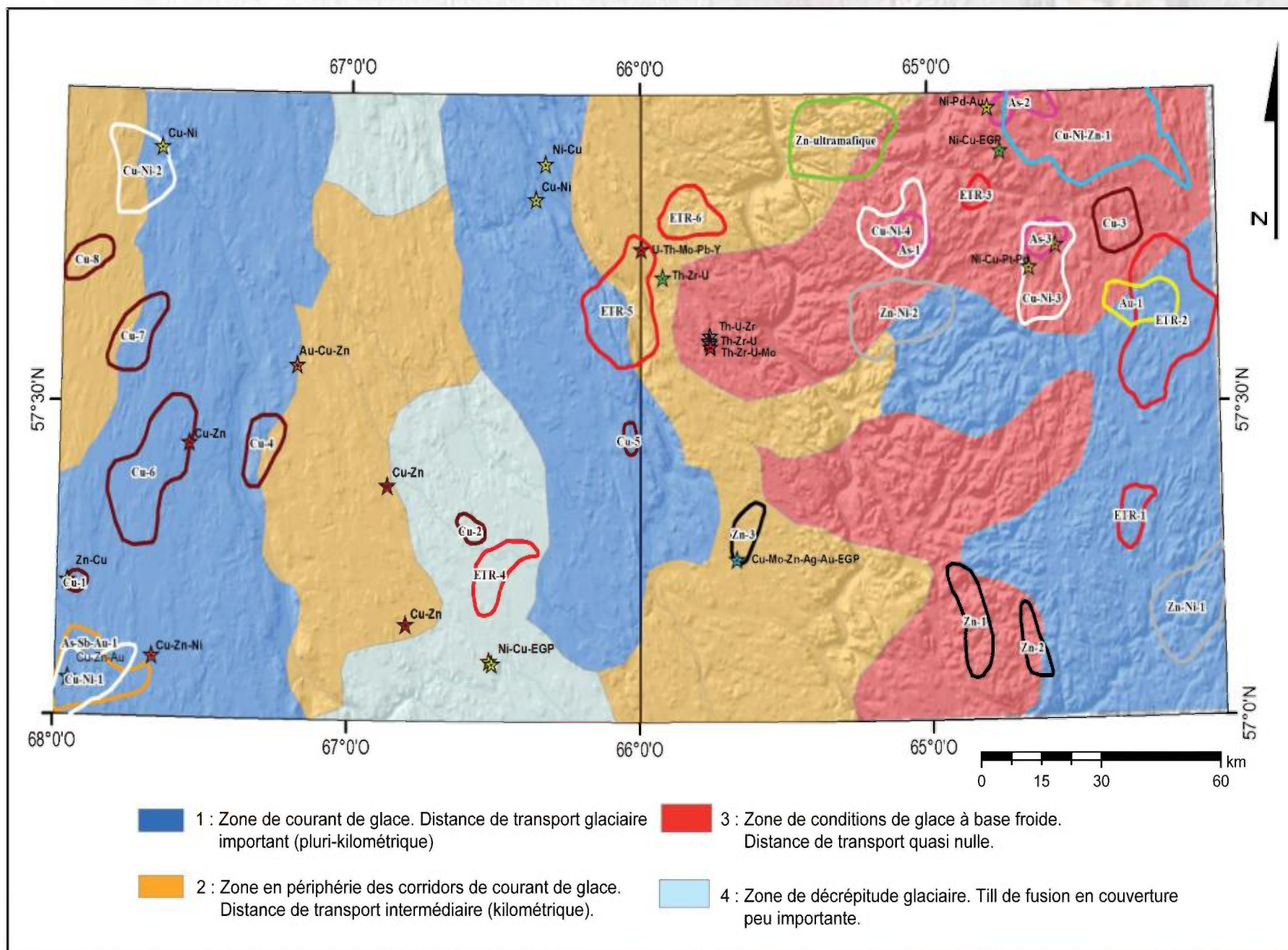
FIGURE 3 – Mosaïque des conditions sous-glaciaires et des distances de transport relatives associées.
