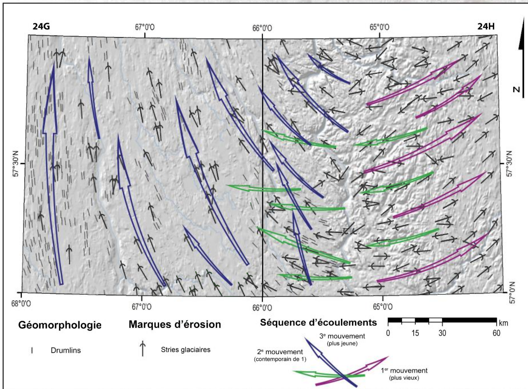
FIGURE 2 – Succession et chronologie relative des mouvements glaciaires récents de la zone d'étude. L'extension des différents mouvements est soulignée par la longueur des flèches.
