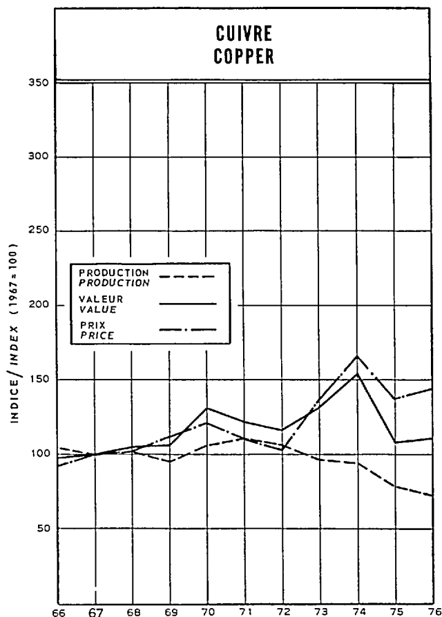
Fig. 6 Indices de la production de cuivre, 1966-1976. Indices of copper production, 1966-1976.
