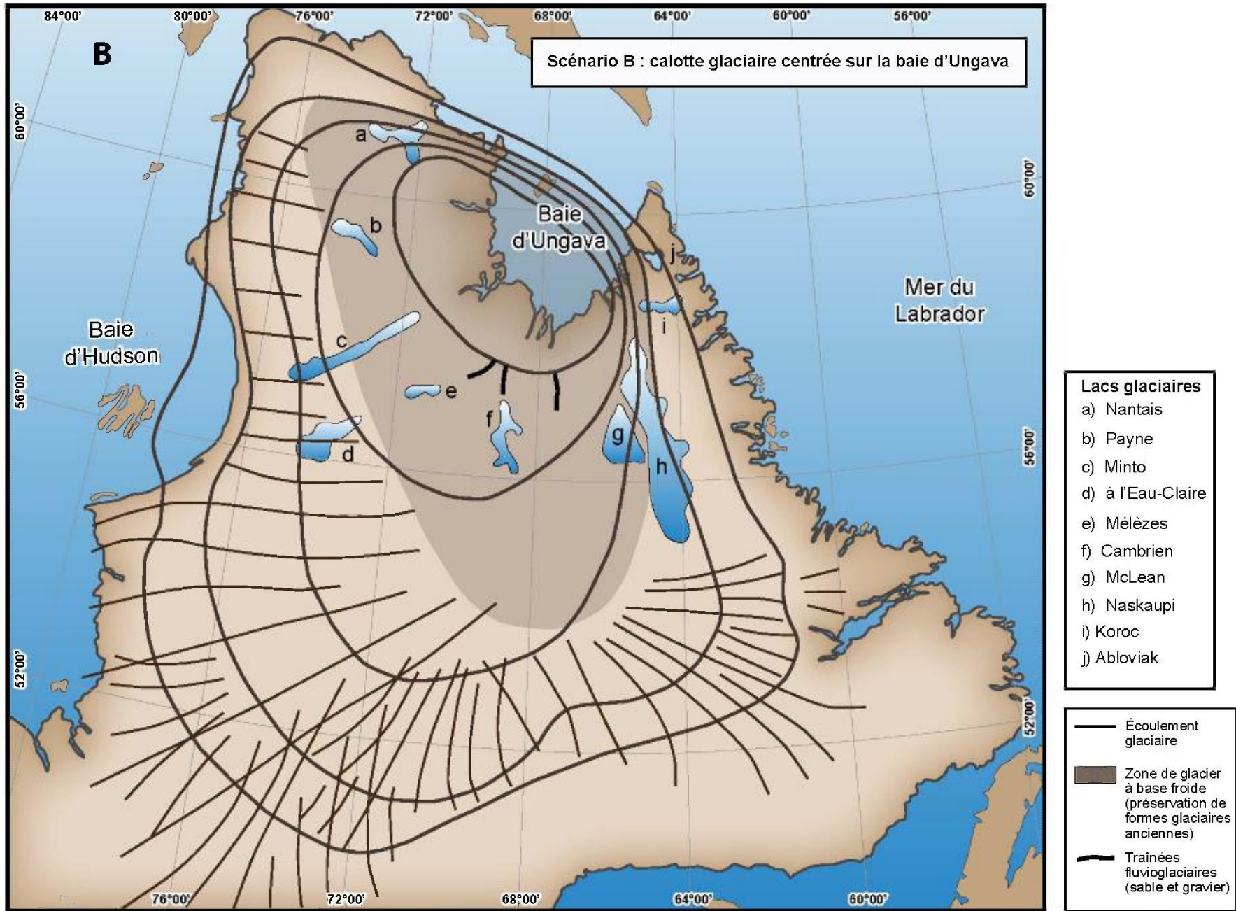
FIGURE 7B – Les formes situées au nord de la ligne de « Horseshoe unconformity » seraient des reliques ayant été préservées sous des conditions de glace à base froide. La limite du « Horseshoe unconformity » correspondrait à la ligne de séparation des ensembles morphosédimentaires d'âge différent (modifiée de Clark et al. , 2000).
