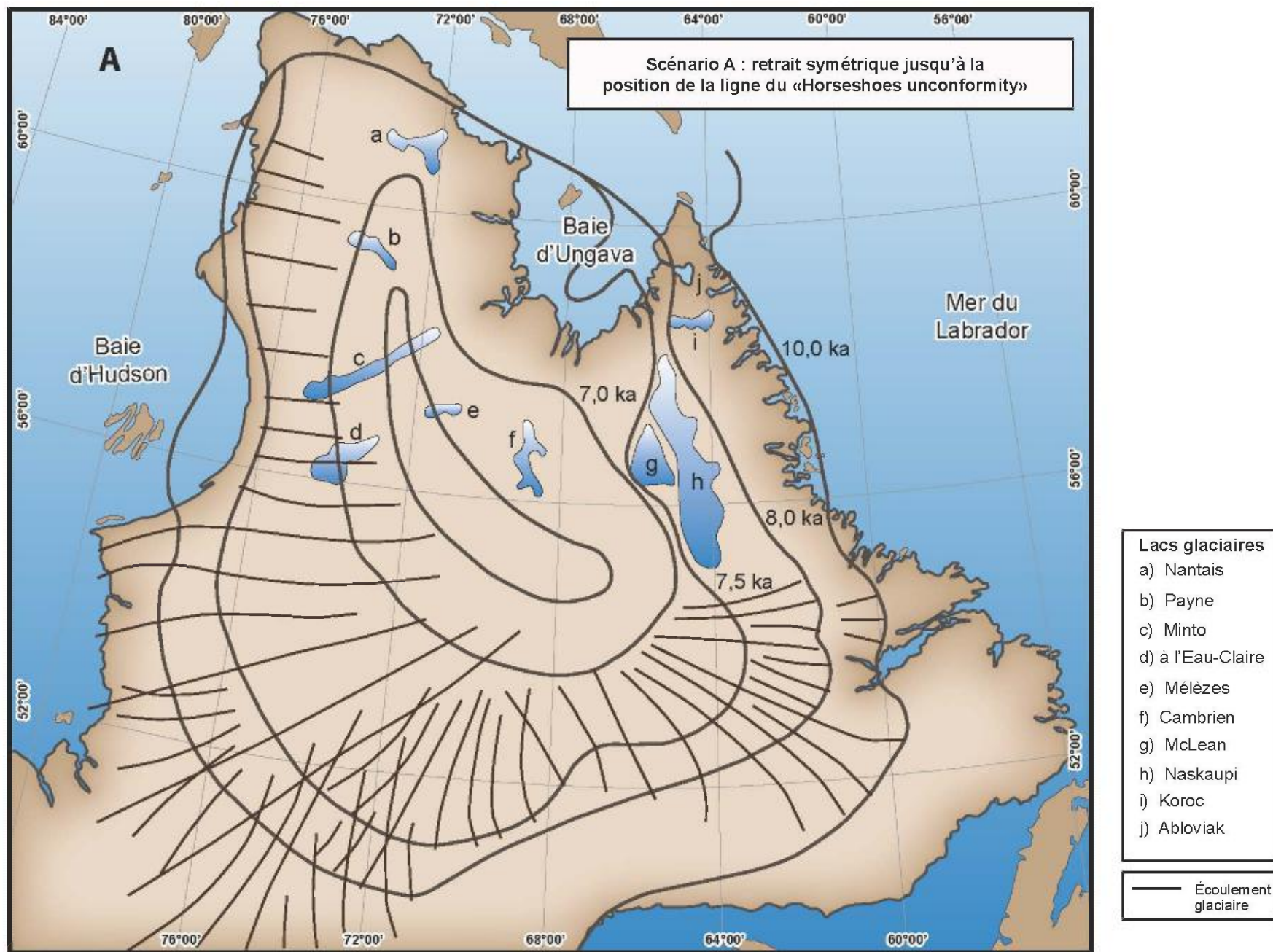
FIGURE 7A – Les formes situées au nord de la ligne de partage glaciaire seraient tardiwisconsinniennes. Le « Horseshoe unconformity » correspondrait à la position tardive de la ligne de partage glaciaire du secteur Labrador-Québec de l'Inlandsis laurentidien.
