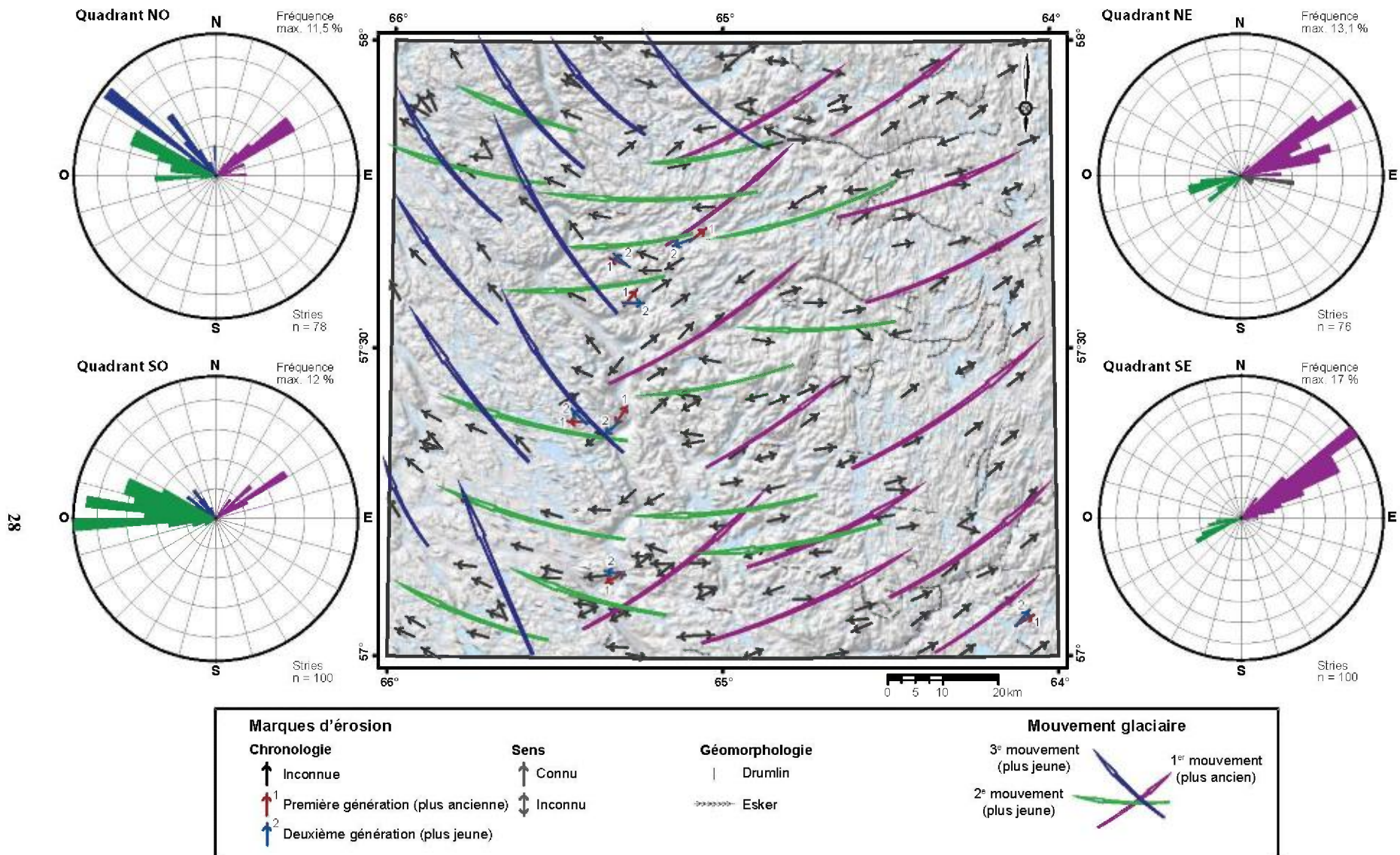
FIGURE 8 – Répartition des marques d'érosion glaciaire mesurées dans la zone d'étude et extension des différents mouvements associés.
