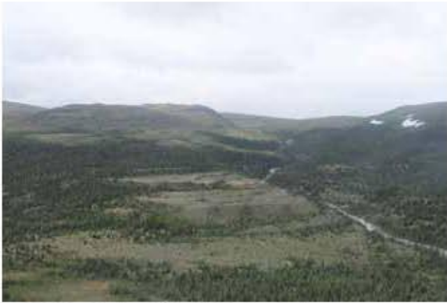
PHOT O 6 – Delta étagé du lac Naskaupi sur la rive ouest de la rivière George.
