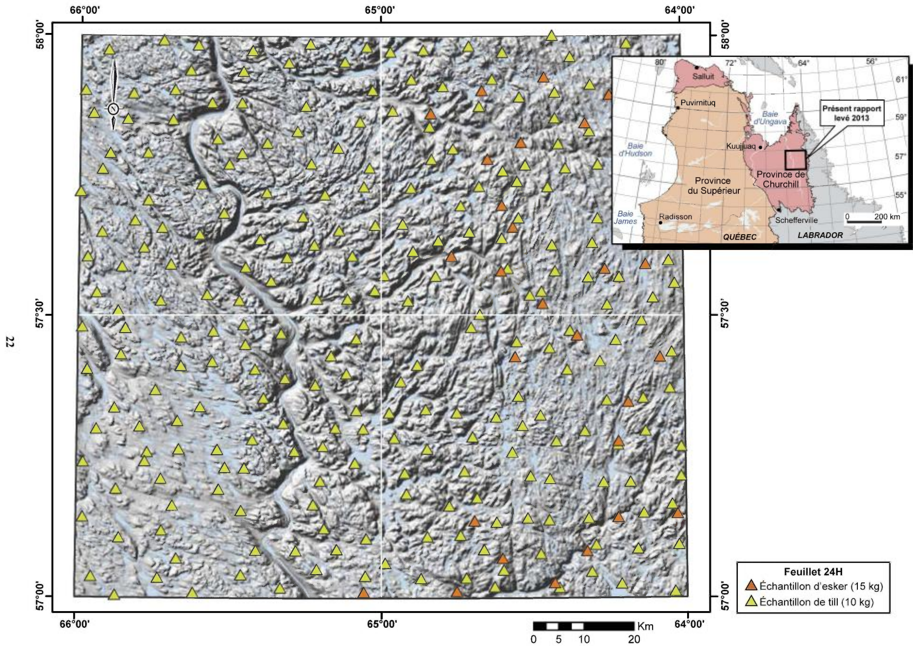
FIGURE 3 – Localisation des échantillons de till et d'esker prélevés au cours de la campagne de terrain 2013.
