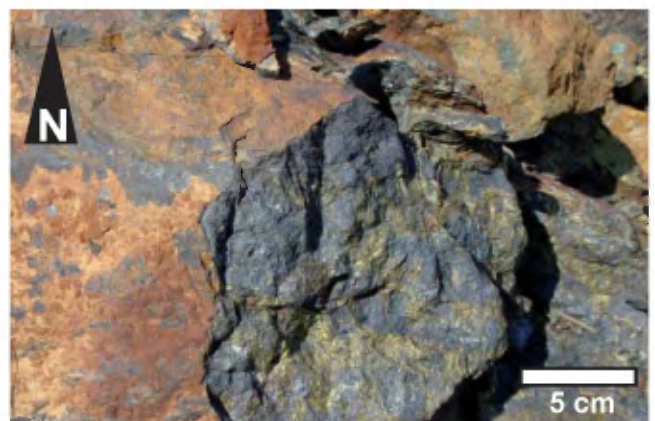
PHOTO 6 - Section très riche en chalcopryrite et magnétite de la veine n°2 de la mine Springer, encaissée dans le Filon-couche de Ventures, à Chapais. Affleurement 09-FL-9375, sur le site de l'ancienne mine Springer.
