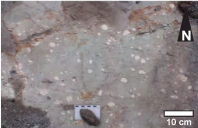
PHOTO 1 - Basalte à phénocristaux glomérophyriques de plagioclase. Membre médian de la Formation d'Obatogamau (Aob), affleurement 09-FL-9008, au sud de la route 113 à l'est de Chapais.
