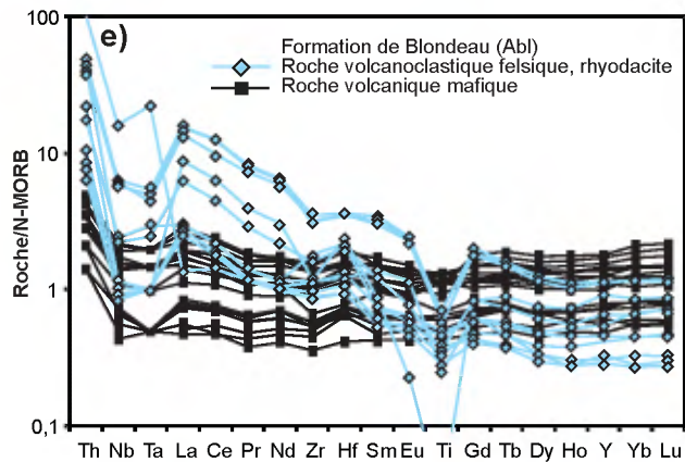
FIGURE 3 - Diagrammes géochimiques des roches volcaniques du Groupe de Roy : a) modifié de Winchester et Floyd, 1977; b) modifié de Ross et Bédard, 2009. Diagrammes des éléments traces pour : c) les roches volcaniques des formations de Chrissie (Acs) et d'Obatogamau (Aob); d) les roches volcanoclastiques et volcaniques felsiques de la Formation de Waconichi (Awa); e) les roches volcanoclastiques felsiques, rhyodacite et volcaniques mafiques de la Formation de Blondeau (Abl); f) les filons-couches de Ventures (Aven) et de Bourbeau (Abou). Normalisation au N-MORB selon les données de Klein (2004).
