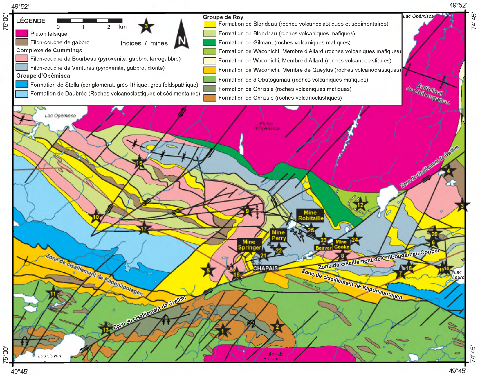
FIGURE 4 - Géologie simplifiée de la région de Chapais (SNRC 32G15-200-0101) et localisation des indices mentionnés dans le présent rapport et listés dans le tableau 1.
