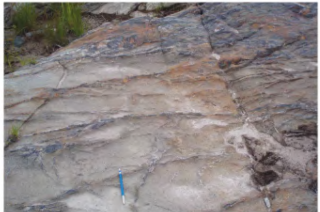
PHOTO 4 - Minéralisation de type porphyrique dans une diorite appartenant à l'Intrusion de Ell. La diorite est recoupée par un stockwerk de veines à tourmaline, quartz, grenat, chalcopryrite, pyrrhotite et pyrite.
