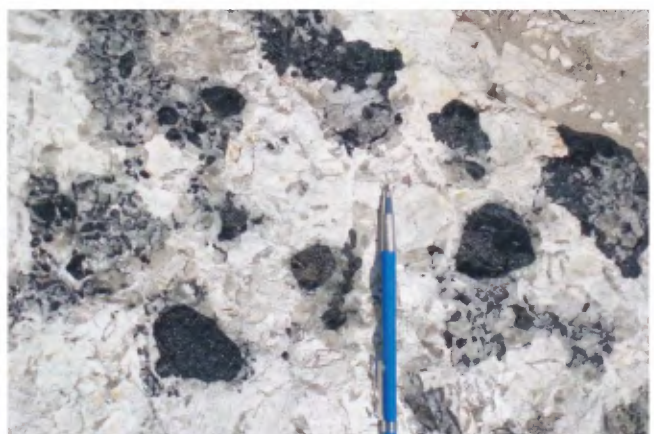
PHOTO 6 - Pegmatite blanche à tourmaline localisée à la limite entre les sous-provinces de La Grande et d'Opinaca.
