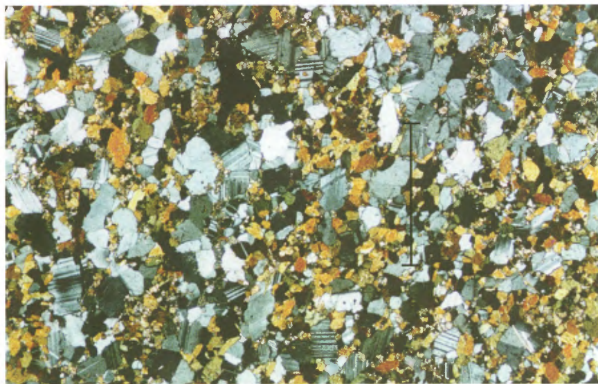
FIGURE 9 - Gabbro à grains fins et frais provenant de l'affleurement 96-2049 et observé sous lumière polarisée. Le trait sur la photo mesure 1,25 mm.
