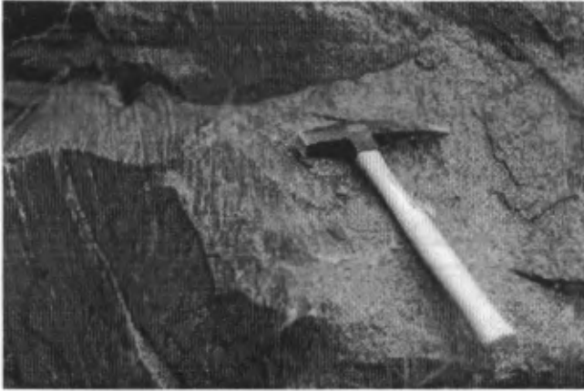
FIGURE 6 - Faciès très écrasé du Granite de La Baie (mPlba) dans lequel les phénocristaux de feldspaths sont étirés comme des rubans. Affleurement 96-1112.
