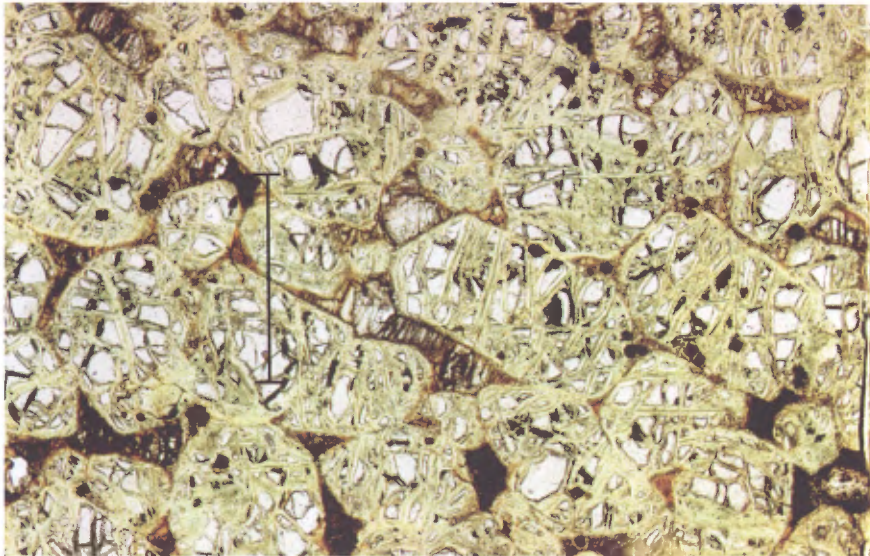
FIGURE 2 - Grains d'olivine partiellement serpentinisés et peu déformés de la Suite mafique-ultramafique de la Baie à Cadie (mPcad). La lame mince de l'échantillon provenant de l'affleurement 96-4010 est éclairée sous lumière naturelle. Le trait sur la photo mesure 1,25 mm.
