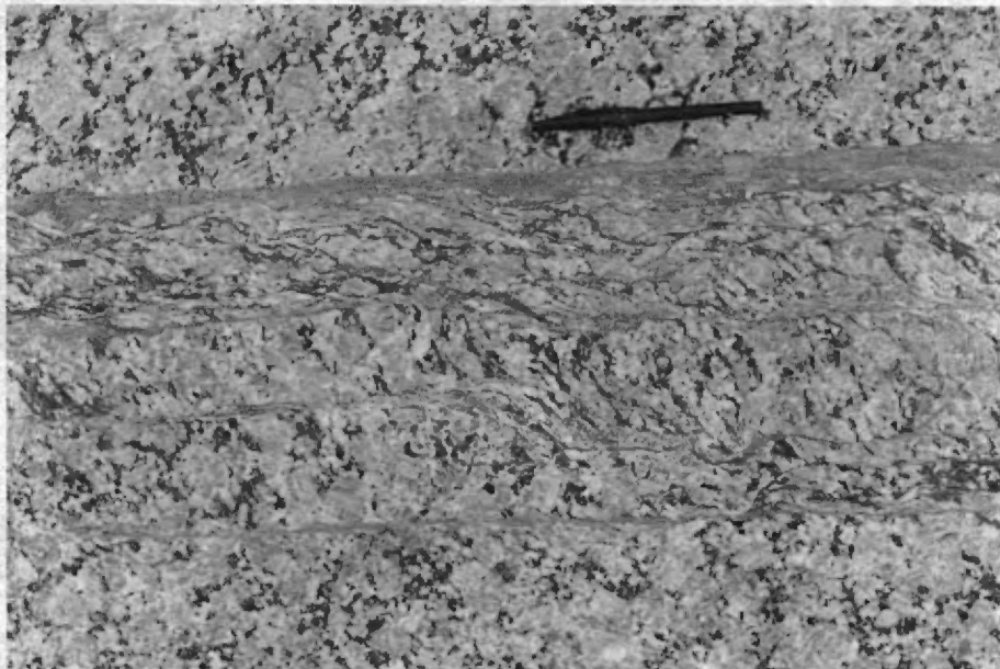
Déformation senestre dans la Mangérite de Pikauba. ( Affleurement 96-1026 )
