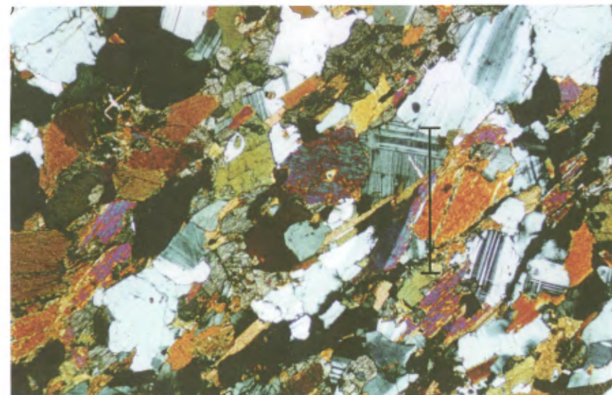
FIGURE 10 - Gabbro à grains grossiers provenant de l'affleurement 96-1029 et observé sous lumière polarisée. Le trait sur la photo mesure 1,25 mm.
