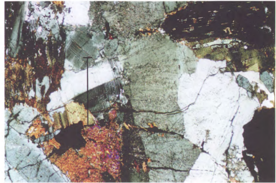
FIGURE 3 - Phénocristaux craquelés et disloqués de plagioclase et des traces de pyroxènes partiellement amphibolitisés et biotitisés observés dans la lame mince, sous lumière polarisée, d'un échantillon provenant de l'affleurement 96-1004 dans la Suite anorthositique de Lac-Saint-Jean (mPlsj). Le trait sur la photo mesure 1,25 mm.
