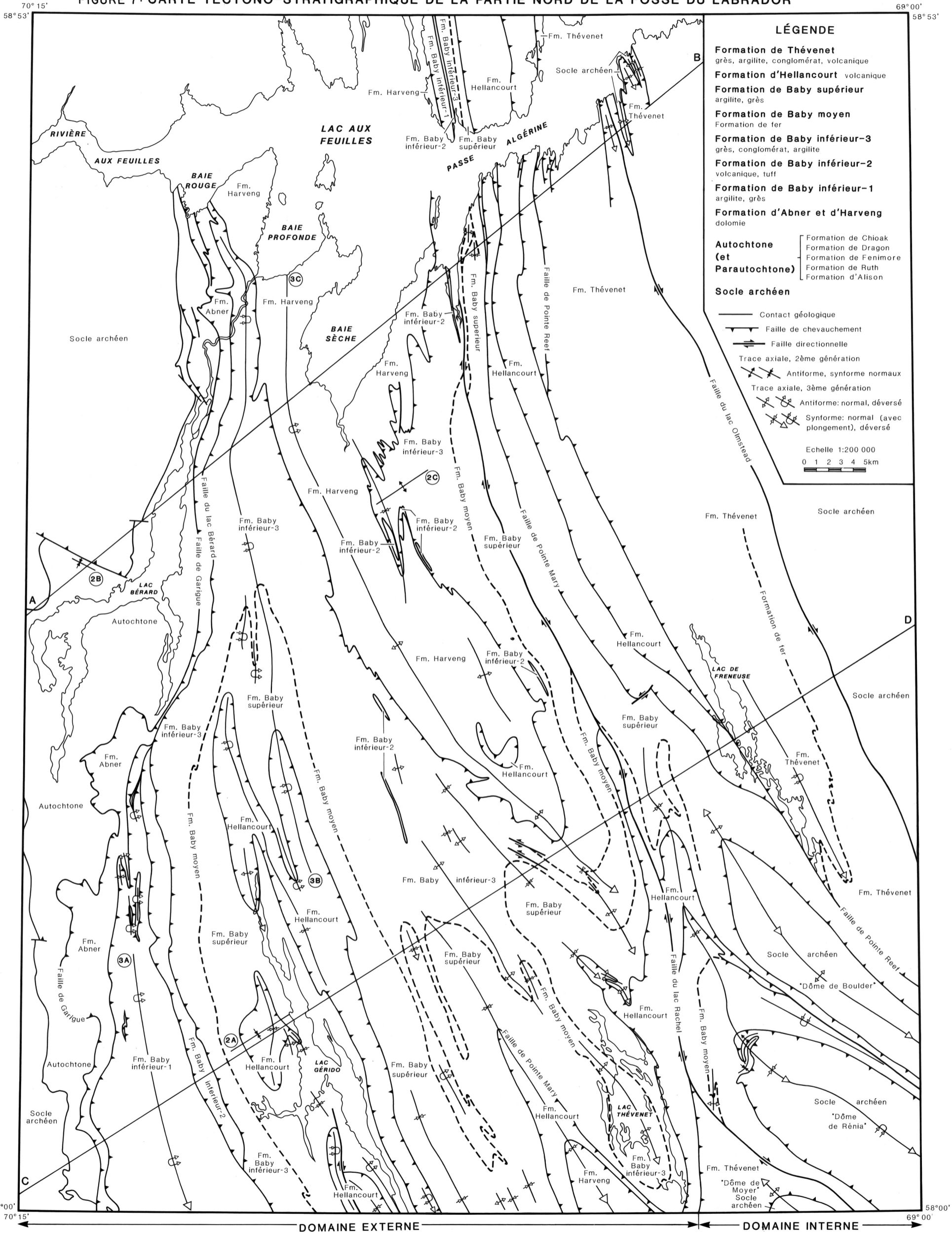
FIGURE 7: CARTE TECTONO-STRATIGRAPHIQUE DE LA PARTIE NORD DE LA FOSSE DU LABRADOR
