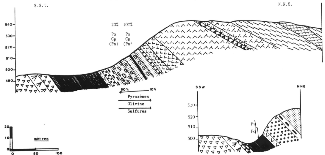
COUPE 2: LAC CHANCE (SUD)
