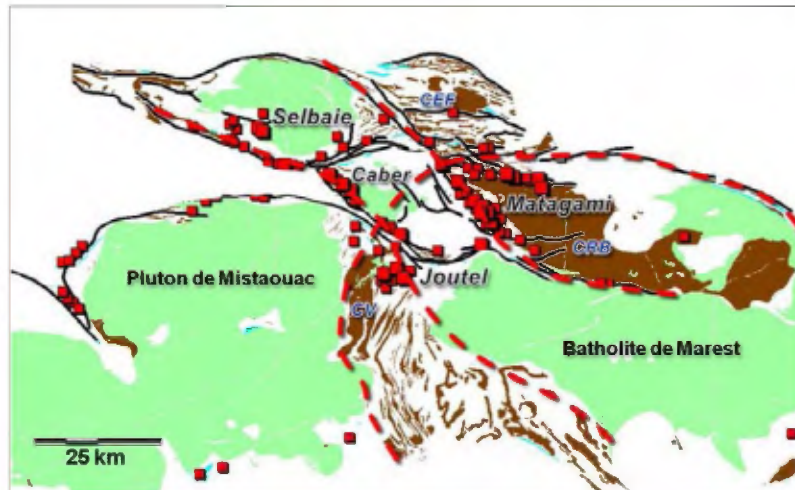
Figure 18. Scénario II de reconstitution paléogéographique de l'arc volcanique du NO de l'Abitibi, camps miniers de Matagami, Selbaie et Joutel. A) retrait du Bassin sédimentaire de Taïbi (2697-2685 Ma) et des volcanites de Cartwright (2721 Ma); B). Références sur les dates dans le texte. C) CRB; complexe de la Rivière-Bell, CV; Complexe de Valrennes, CEF; Complexe d'Enjalran-Fenelon. Pour plus de détail se référer au texte.
