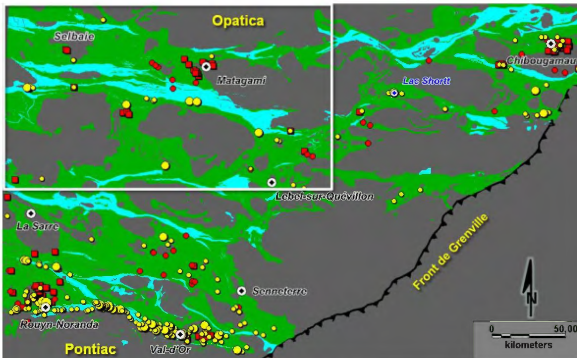
Figure 1. Localisation de la région d'étude (encadré blanc) dans la Sous-province d'Abitibi. Carte géologique selon SIGEOM (2007).
