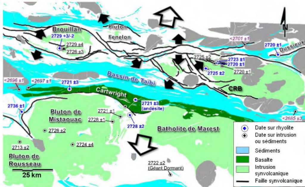
Figure 16. Principaux bassins sédimentaires (cyan) et intrusions synvolcaniques (vert clair) avec les directions inférées d'extension régionale et locale. Les dates en noir (en Ma) proviennent d'intrusions. Les dates en mauve proviennent de roches sédimentaires (signe <) et celles en bleu de roches volcaniques. Dates d'après la compilation de Goutier et Melançon (2010). Les plutons en gris sont syn ou post-tectoniques.
