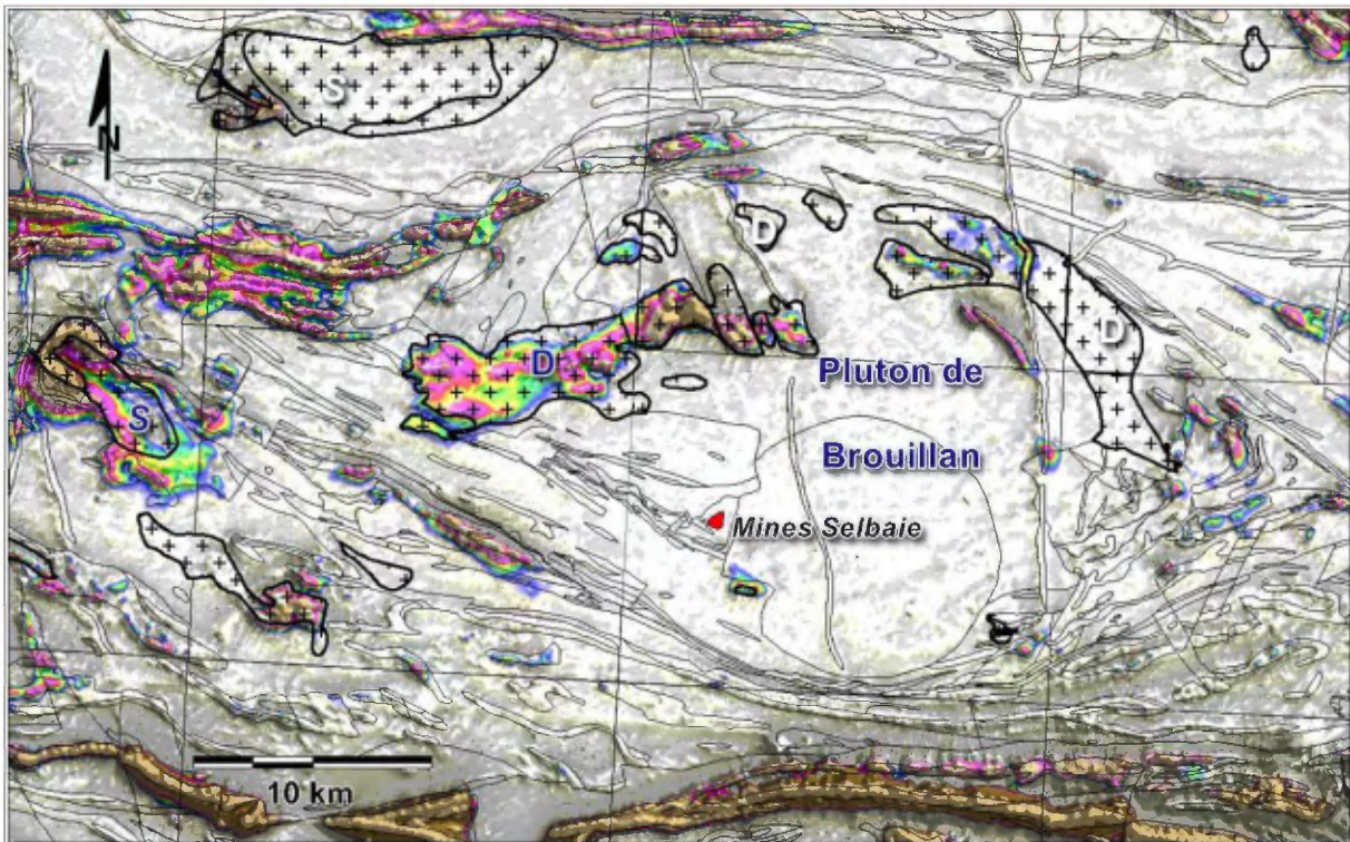
Figure 13. Champ magnétique total (MEGATEM de Xstrata Zinc) en couleurs et en transparence sur la première dérivée verticale du champ total en tons de gris et ombragé de la région des Mines Selbaie montrant la signature magnétique des diorites synvolcaniques (D) et des intrusions syntectoniques (S).
