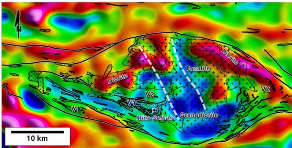
Figure 14. Gradient vertical du levé gravimétrique hélicoptéré (DP 2008-02) montrant le principal bassin interprété de rhyolites (V1) à l'ouest des Mines Selbaie et l'enracinement de la granodiorite subcirculaire et une structure de graben orientée NNO sous les intrusions synvolcanique de Brouillan recoupant les diorites (traits blancs). V2; andésite. Les fortes anomalies gravimétriques sont de couleur mauve et les faibles sont de couleur cyan à bleu.
