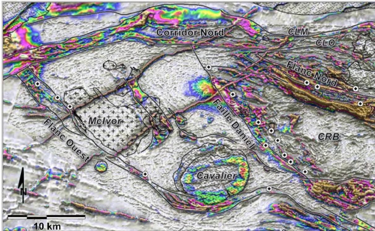
Figure 10. Champ magnétique total en couleurs et en transparence sur la première dérivée verticale du champ total en tons de gris et ombragée avec les principales limites (lignes noires) de domaines magnétiques. Ces limites sont interprétées comme des failles synvolcaniques. Les ronds blancs avec un losange noir indiquent l'emplacement des dépôts de SMV. CLM : cisaillement du Lac Matagami, CLO : cisaillement Lac Olga.
