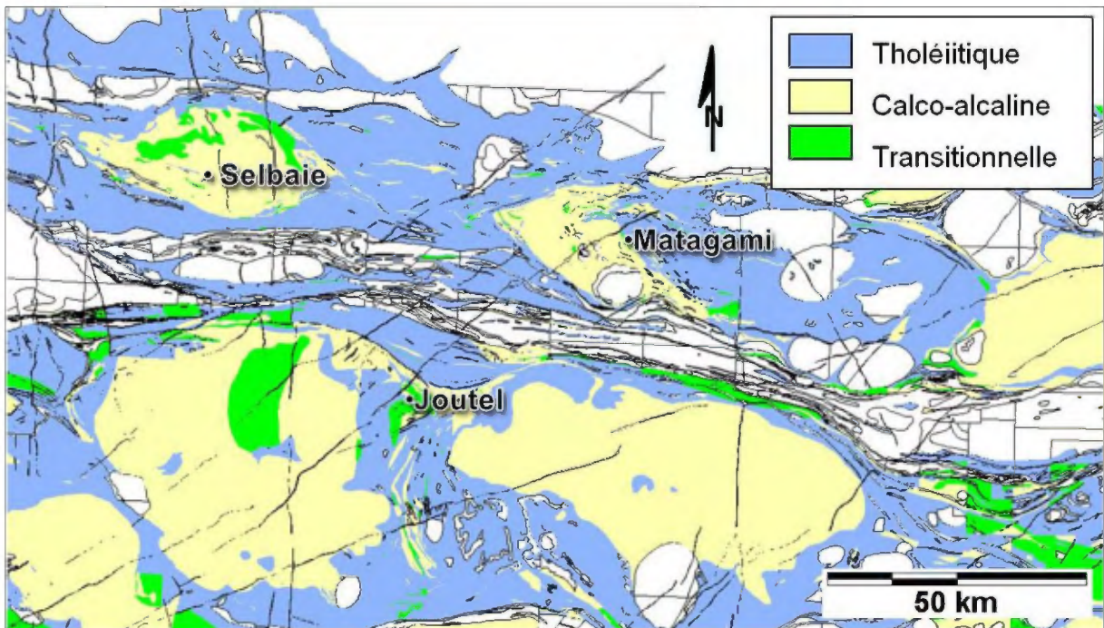
Figure 4. Carte des affinités géochimiques selon la classification de Barrett et MacClean (1994) des roches volcaniques intrusives et extrusives du NO de l'Abitibi. Les régions laissées en blanc représentent des intrusions orogéniques ou ultramafiques, ou des bassins métasédimentaires.
