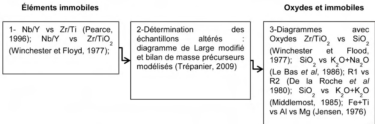
Figure 3. Cheminement et diagrammes utilisés pour classer les échantillons lithogéochimiques, de rhyolite à basalte.
