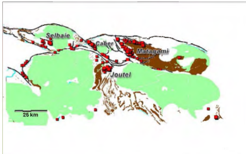
Figure 17. Scénario I de reconstitution paléo-tectonique de l'arc volcanique du NO de l'Abitibi, camps miniers de Matagami, Selbaie et Joutel sans aucune modification des polygones de la carte géologique. A) Retrait du Bassin sédimentaire de Taïbi (2697- 2685 Ma) et des volcanites de Cartwright (2721 Ma), gabbros (en brun); B) Références sur les dates dans le texte.
