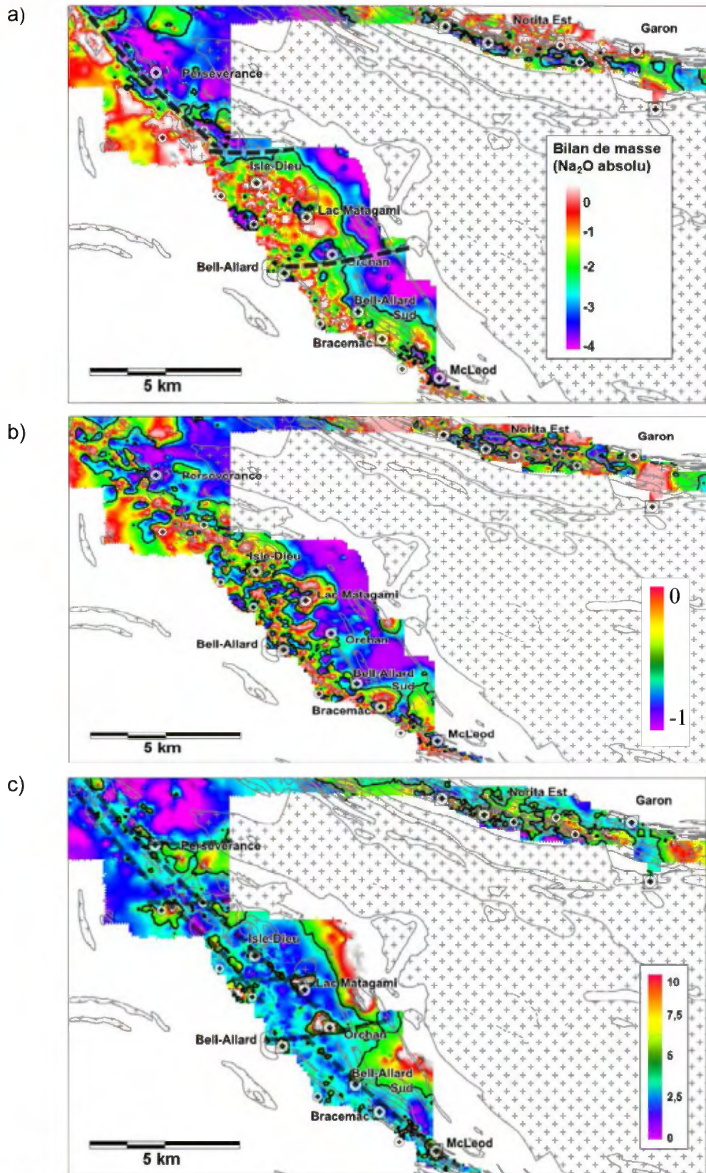
Figure 8. Bilan de masse absolue calculé à partir de précurseurs modélisés (Trépanier, 2009) pour le Camp minier de Matagami. A) Na 2 O, B) K 2 O et C) Fe 2 O 3 total. Les valeurs sur la barre de couleurs représentent les gains (+) et pertes (-) de masse en g/100g. Traits noirs représentent la trace de failles synvolcaniques interprétées.
