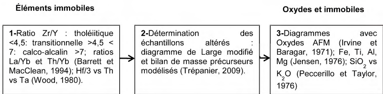
Figure 2. Cheminement, critères et diagrammes utilisés pour discriminer l'affinité géochimique des échantillons lithogéochimiques (tholéitique, transitionnel et calco-alkalin).
