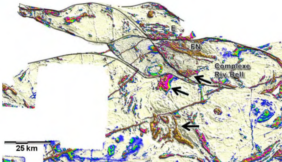
Figure 19. Signature magnétique selon l'état final du scénario de reconstitution II montrant la similitude des anomalies magnétiques entre le Complexe d'Enjalran-Fenelon (E) et le flanc Nord (FN) de Matagami. Noter la continuité magnétique vers l'ouest et ensuite vers le sud de l'anomalie magnétique située dans le sud du Complexe de la Rivière Bell (CRB) et indiquée par les trois flèches noires.
