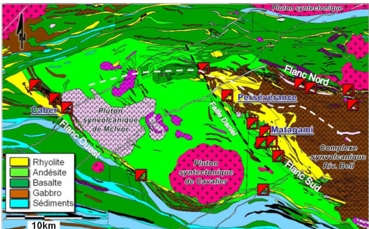
Figure 5. Carte géologique du Camp minier de Matagami (modifiée du Sigeom 2009, Xstrata Zinc, cette étude) montrant la distribution des gisements de sulfures massifs volcanogènes (carrés rouges). Les tirets blancs représentent la trace axiale interprétée de l'Anticlinal de Galinée.
