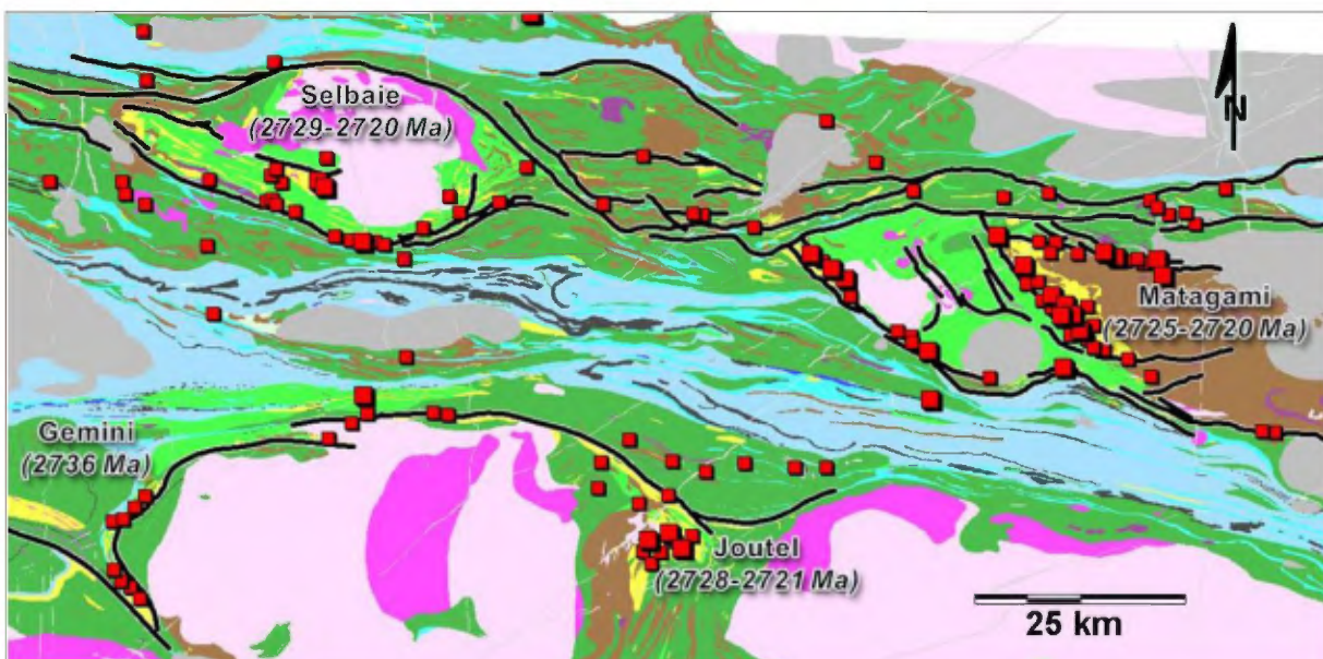
Figure 15. Carte géologique du NO de l'Abitibi avec les failles synvolcaniques proposées (trait gras noir). Dates d'après la compilation de Goutier et Melançon (2010). Même légende géologique que la Figure 11. Plutons en tons de rose; rose pâle (felsiques), rose foncé (intermédiaire). Plutons en gris représentent des intrusions syn ou post-tectoniques. Gisements (gros carré rouge) et gîtes (petit carré rouge) de Zn et/ou Cu.
