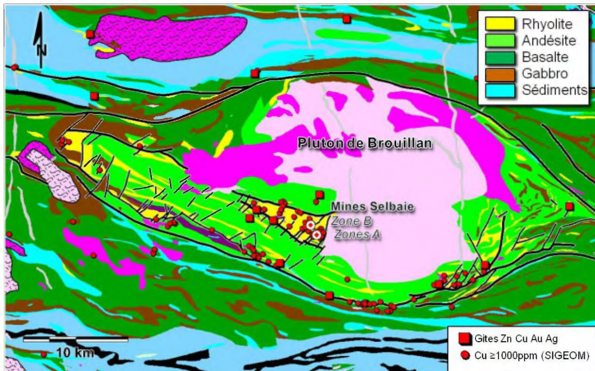
Figure 12. Carte géologique de la région des Mines Selbaie (modifiée du SIGEOM 2009). Plutons en tons de rose; rose pâle (felsiques) rose foncé (intermédiaire). Les plutons avec une trame de sigmoïdes sont des plutons syn- ou post-tectoniques. Intrusions ultramafiques en mauve foncé.
