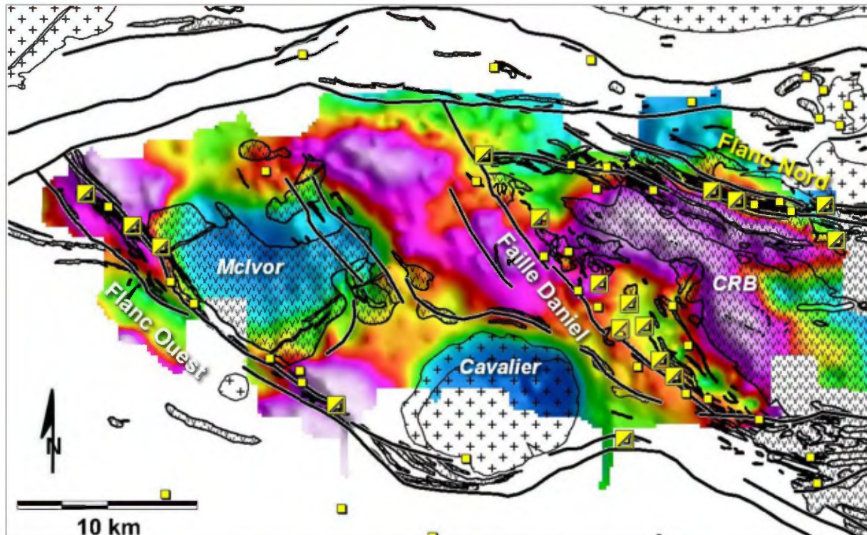
Figure 11. Gravité résiduelle de l'anomalie de Bouguer mesurée au sol pour la région de Matagami (données publiques de Jobin et al. , 2009 et non-publiques de Xstrata Zinc). Les fortes anomalies gravimétriques sont de couleur mauve et les faibles sont de couleur cyan à bleu. Gros carrés jaunes; Gisements de SMV; petits carrés jaunes; gîtes de SMV.
