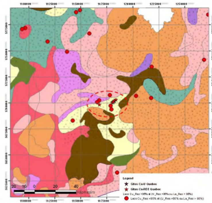
Figure 64: Anomalies en \text{Cu}_{\text{Res}} > 95\% ET ( \text{La}_{\text{Res}} > 95\% OU \text{U}_{\text{Res}} > 95\% ) par régression spatiale, levé 1988050, secteur de Kwyjibo. Retour au texte
