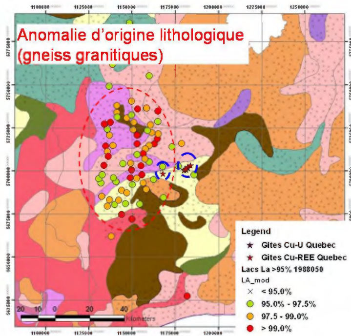
Figure 60: Anomalies en lanthane par les valeurs brutes sur le levé 1988050, secteur de Kwyjibo. Retour au texte
