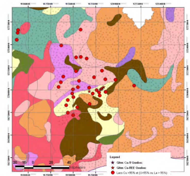
Figure 65: Anomalies en \text{Cu} > 95\% ET ( \text{La} > 95\% OU \text{U} > 95\% ) par les valeurs brutes, levé 1988050, secteur de Kwyjibo. Retour au texte
