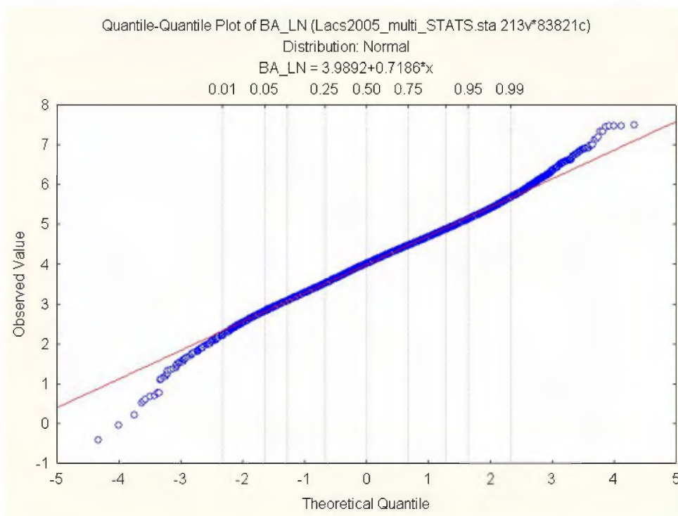
Figure 1: Graphique quantile-quantile pour log(barium) sur l'ensemble du Québec. Retour au texte
