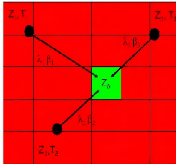
Figure 33: Exemple de cokrigage à deux variables (Z, T) pour évaluer la valeur de Z. Modifié de Yarus et Chambers, 2003. Retour au texte
