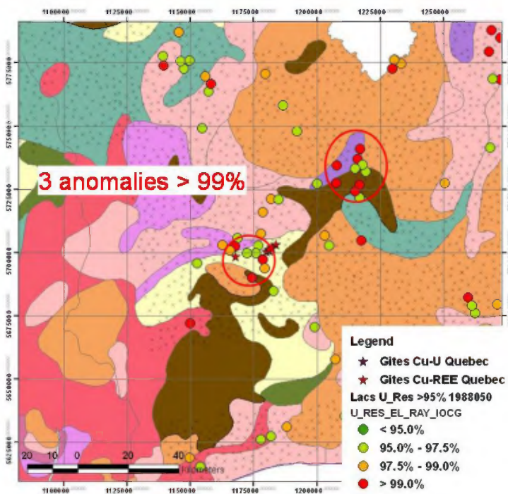
Figure 61. Anomalies en uranium par régression spatiale, levé 1988050, secteur de Kwyjibo. Retour au texte
