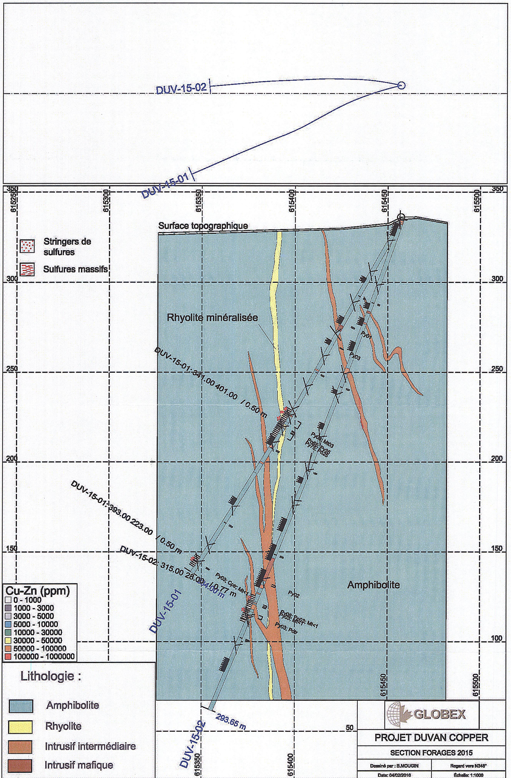
Figure 7 : Section de forage interprétée suite à la campagne 2015
