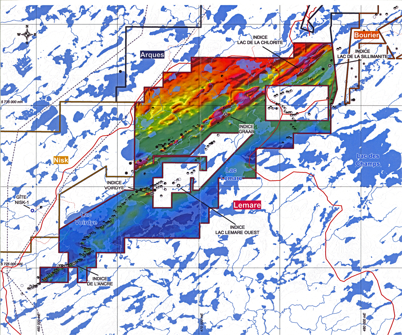
FIGURE 5: CHAMP MAGNÉTIQUE TOTAL ET ANOMALIES TDEM DE LA PROPRIÉTÉ LEMARE
