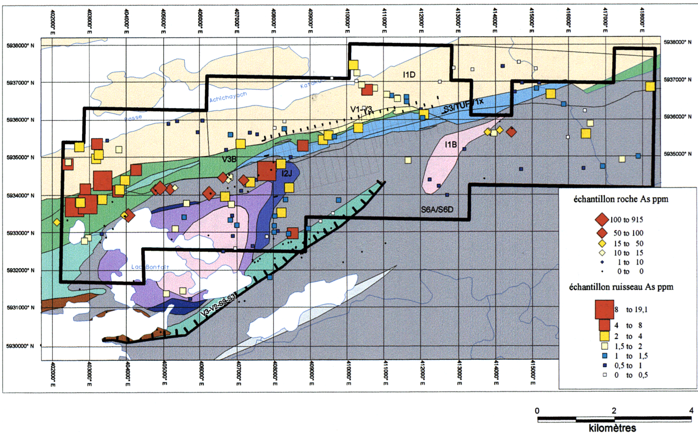
Figure 3 : Carte des anomalies géochimiques Au - Ag - As - Cu
