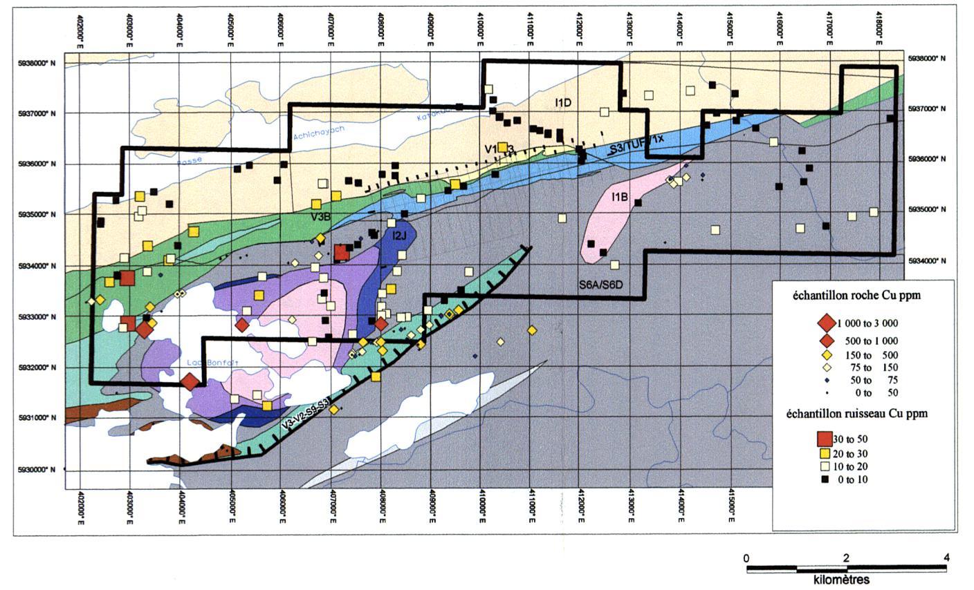
Figure 3 : Carte des anomalies géochimiques Au - Ag - As - Cu
