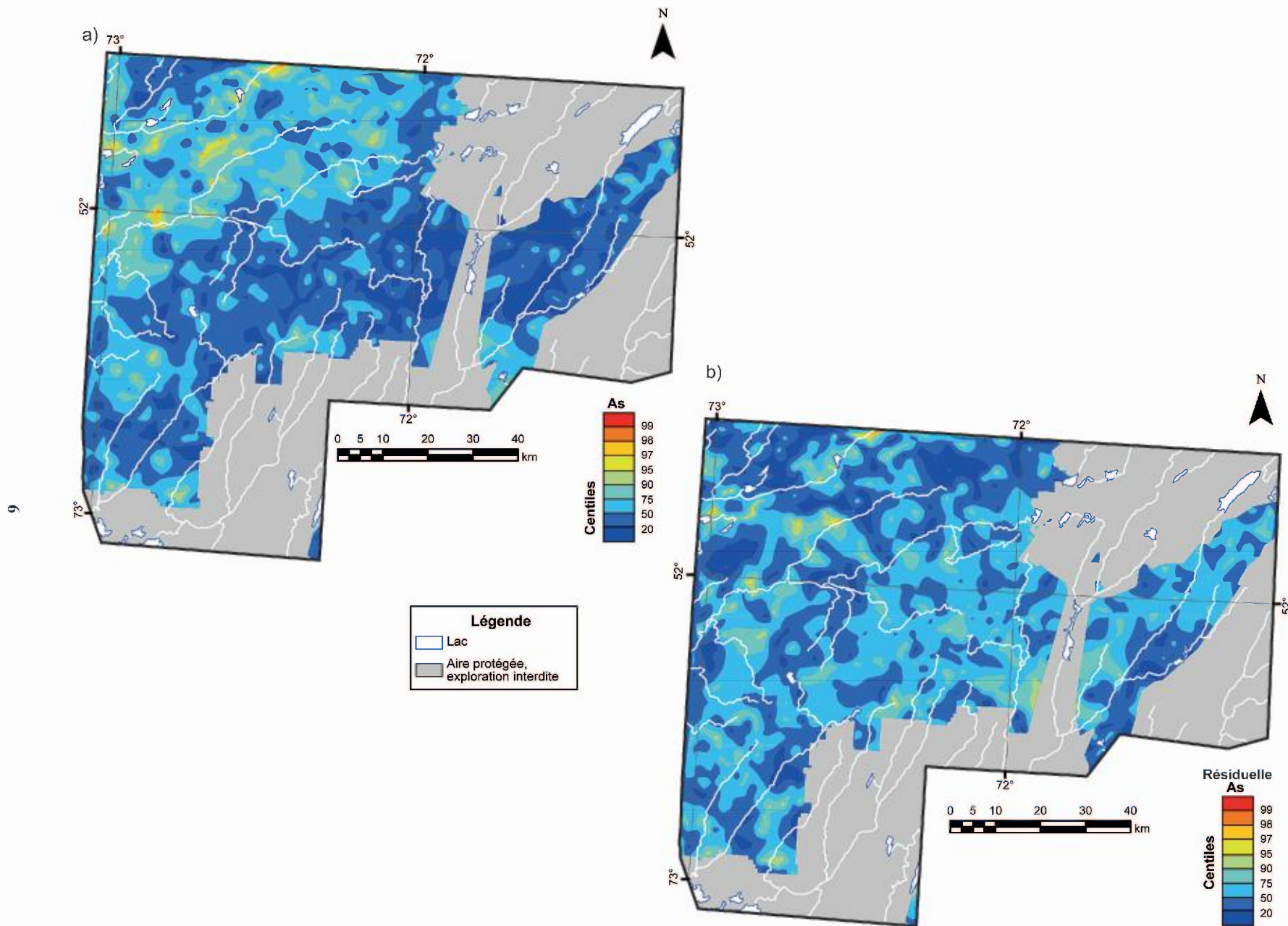
FIGURE 3 – a) Carte des concentrations en As dans les sédiments de fond lac du levé de Mistassini nord. b) Carte des résiduelles après traitement de régression spatiale pour l'arsenic.
