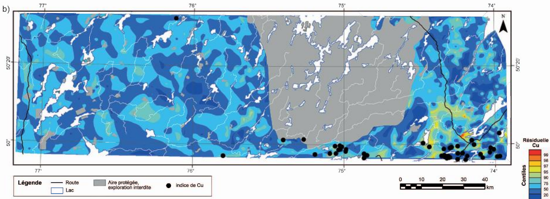
FIGURE 5 – a) Carte des concentrations en Cu dans les sédiments de fond de lac du levé Assinica. b) Carte des valeurs résiduelles après traitement de régression spatiale pour le cuivre.
