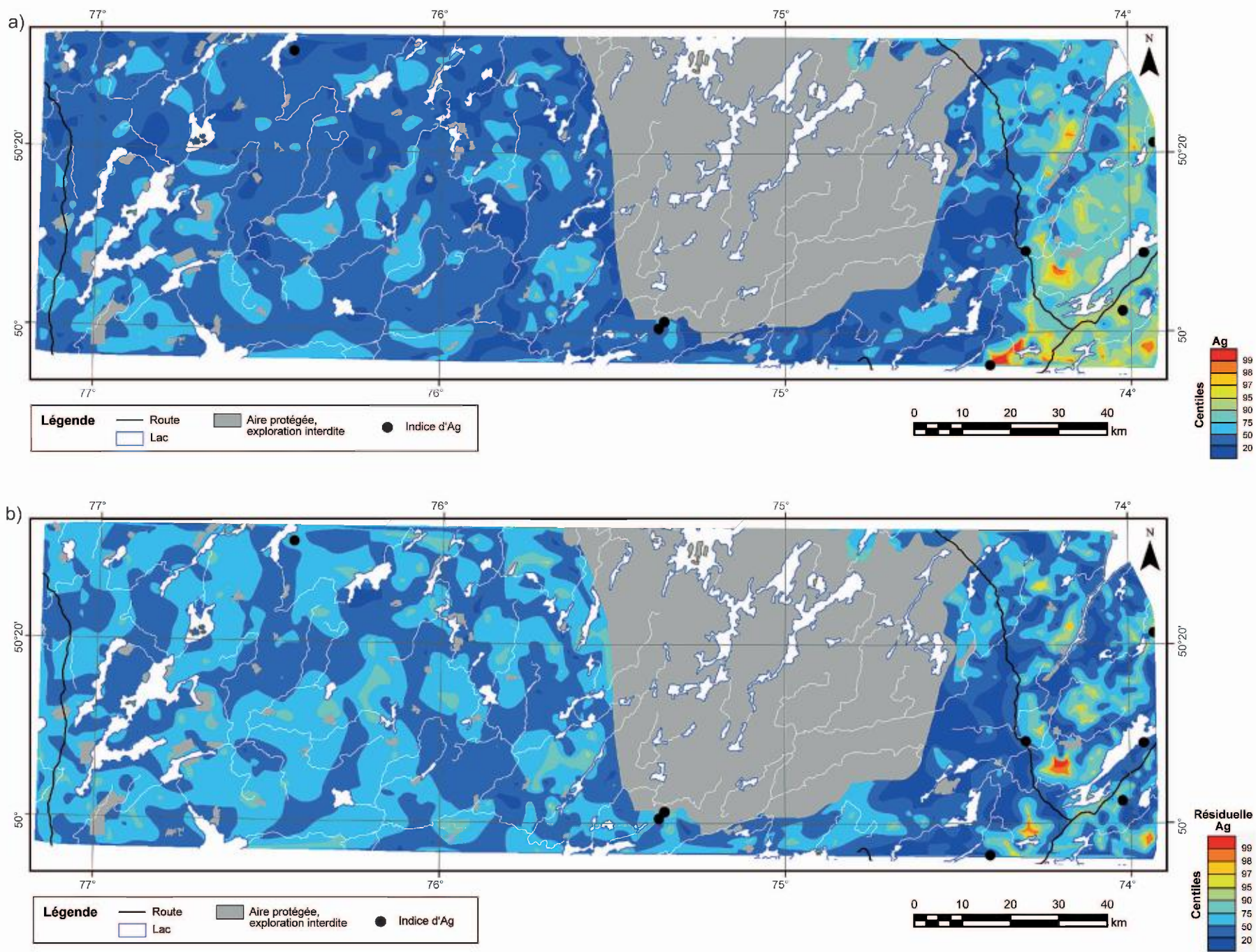
FIGURE 2 – a) Carte des concentrations en Ag dans les sédiments de fond de lac du levé Assinica. b) Carte des valeurs résiduelles après traitement de régression spatiale pour l'argent.
