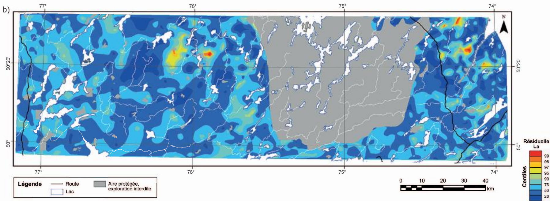
FIGURE 6 – a) Carte des concentrations en La dans les sédiments de fond de lac du levé Assinica. b) Carte des valeurs résiduelles après traitement de régression spatiale pour le lanthane.
