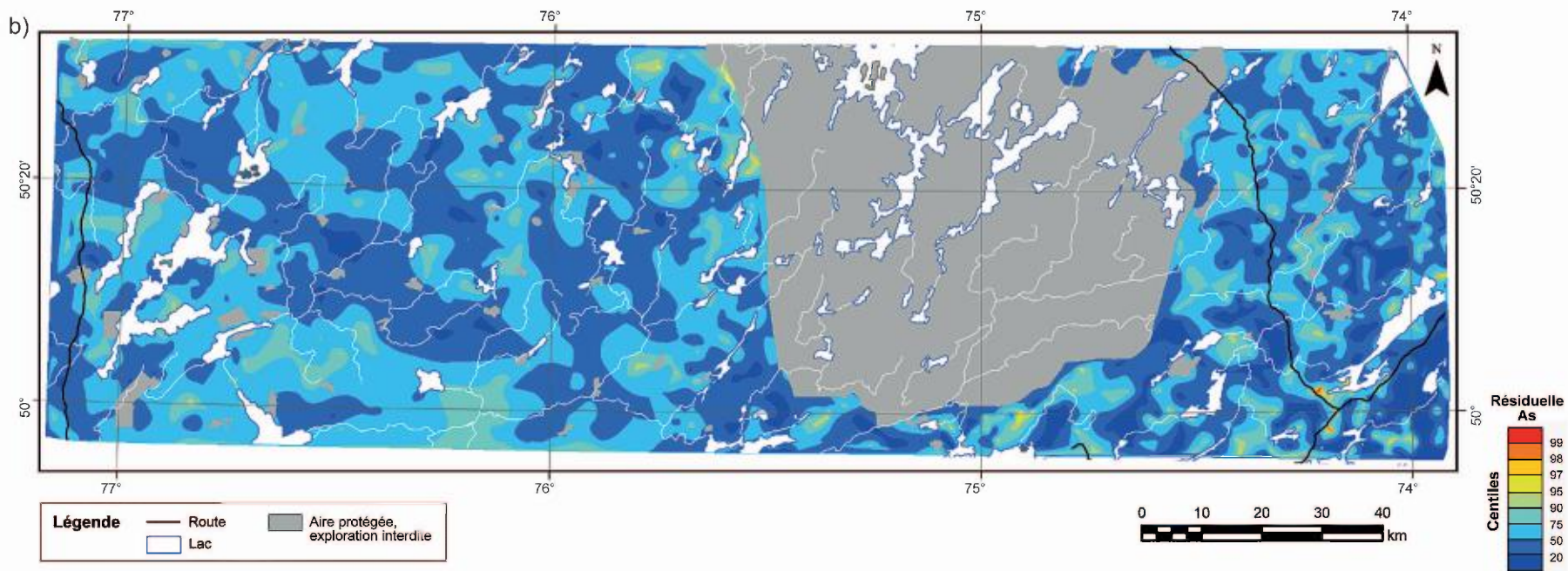
FIGURE 3 – a) Carte des concentrations en As dans les sédiments de fond de lac du levé Assinica. b) Carte des valeurs résiduelles après traitement de régression spatiale pour l'arsenic.
