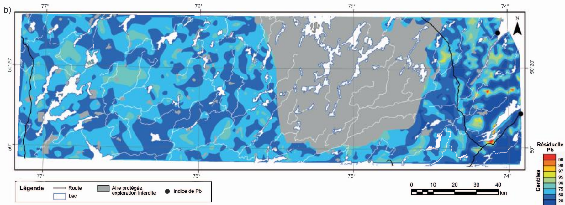
FIGURE 9 – a) Carte des concentrations en Pb dans les sédiments de fond de lac du levé Assinica. b) Carte des valeurs résiduelles après traitement de régression spatiale pour le plomb.
